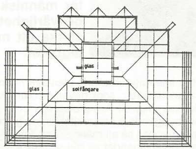
TAKPLAN
