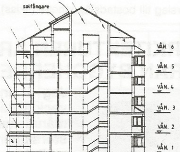
TVÄRSEKTION
