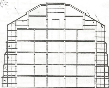
LÄNGDSEKTION
