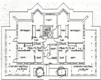
PLAN AV VÅNING 3, 4 OCH 5
