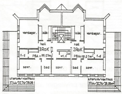
PLAN AV VÅNING 3, 4 OCH 5
