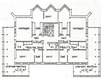
PLAN AV VÅNING 6
