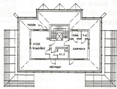
PLAN AV VÅNING 6
