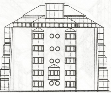
FASAD MOT NORR
