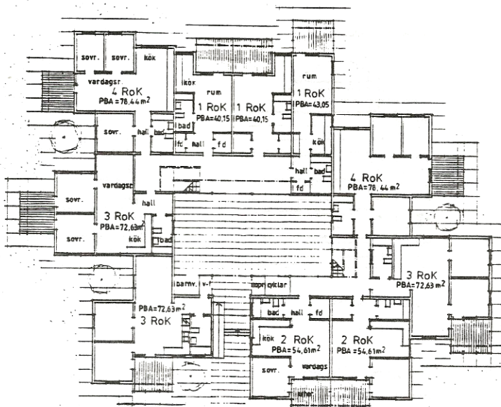
PLAN AV VÅNING 1
